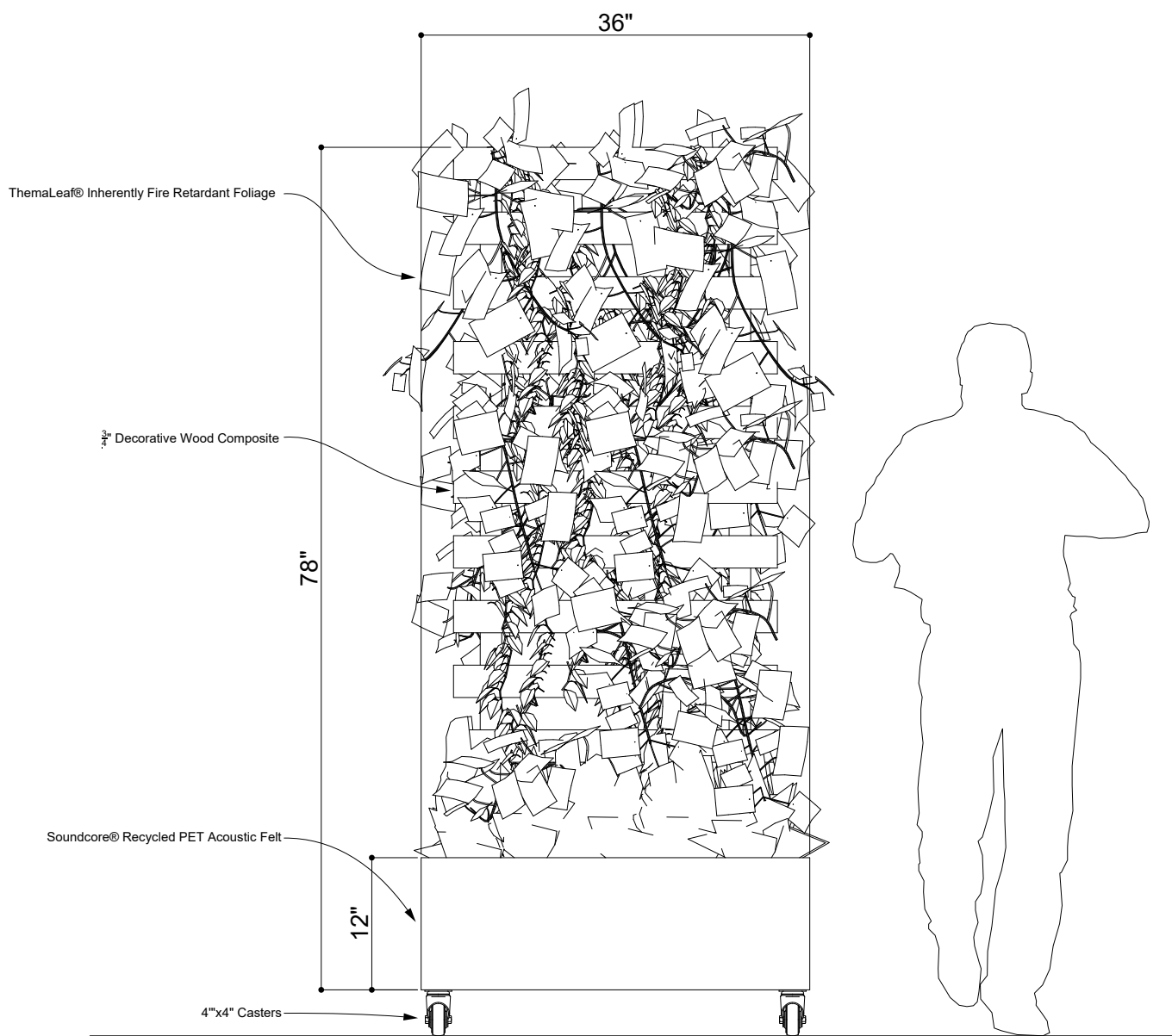
① ELEVATION 1
